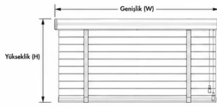
ÖLÇÜLENDİRİLMİŞ GÖRÜNÜŞ
