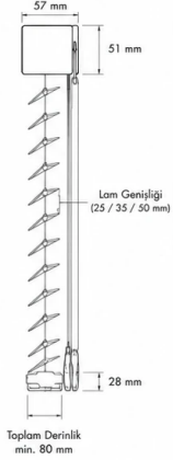
YAN GÖRÜNÜŞ
